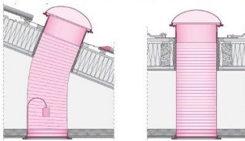
Вертикальное и горизонтальное сечение туннеля дневного света SLT
